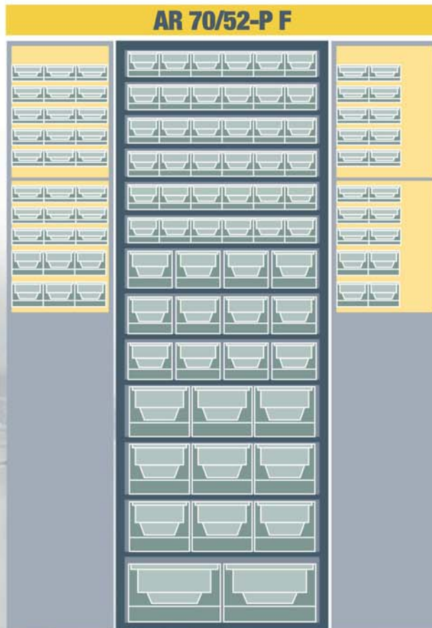
KEY BOX: K1 n. 40 - K2 n. 46 - K3 n. 12 - K4 n. 9 - K5 n. 2 Ripiani / Ledges / Tablettes / Anaqueles / Bretter: n. 16 Pannelli porte / Door panels / Panneaux pour le portes / Paneles por puertas / Türenpanel: n. 4
